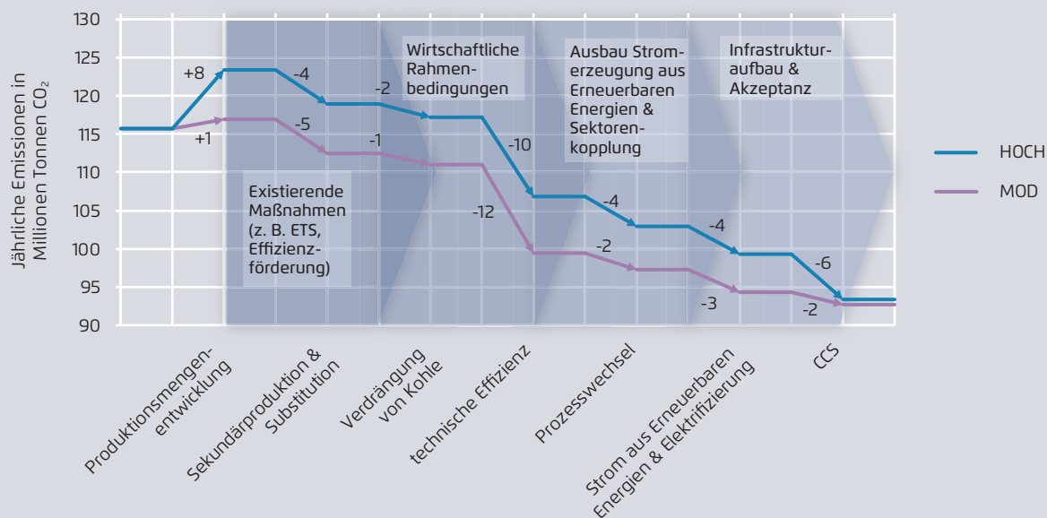
Beiträge der CO 2 -Minderungsstrategien für die Sektoren Stahl, Chemie und Zement sowie die wichtigsten Triebfedern zu ihrer Umsetzung
