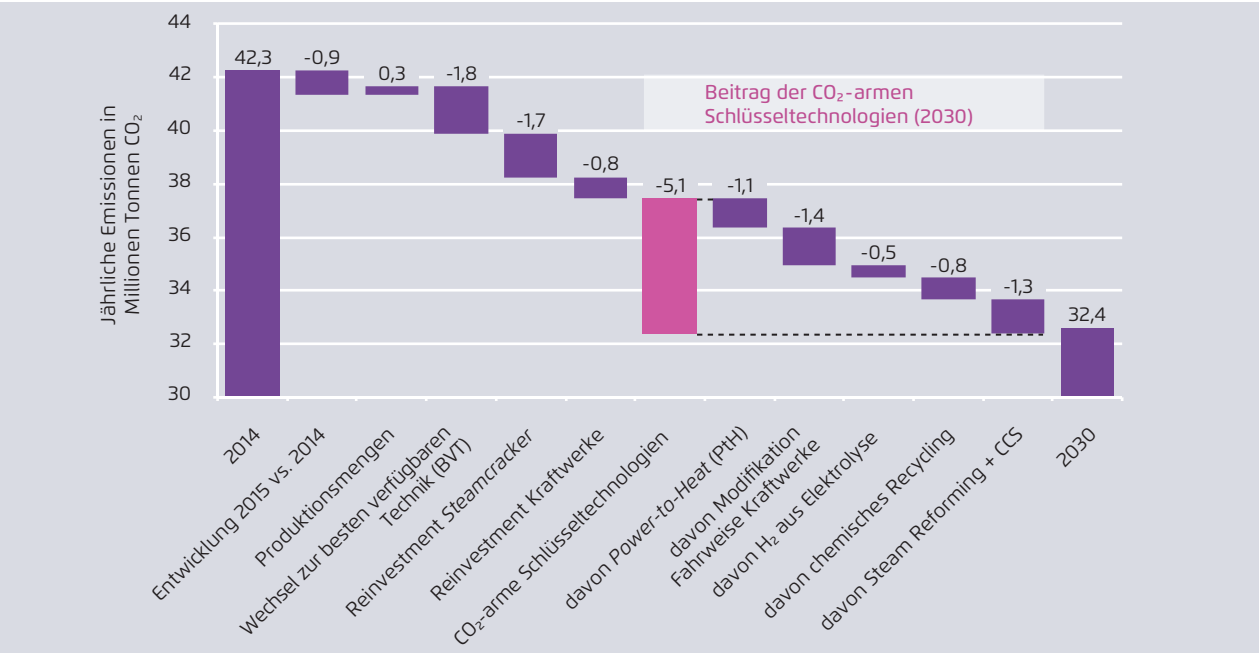
Beiträge der Strategien zur Minderung der direkten Emissionen der chemischen Industrie (Grundstoffe) bis 2030 im Szenario HOCH
